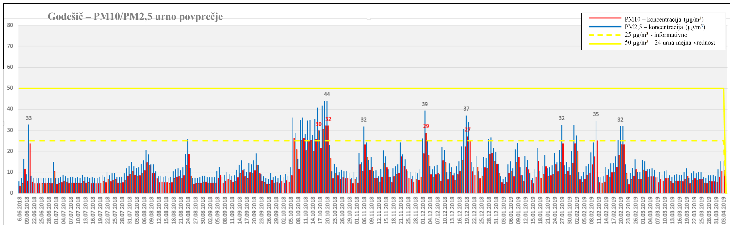
Graf 5: Rezultati meritev PM10 in PM2,5 na merilni postaji GODEŠIČ, v obdobju 01.06.2018 - 30.03.2019
