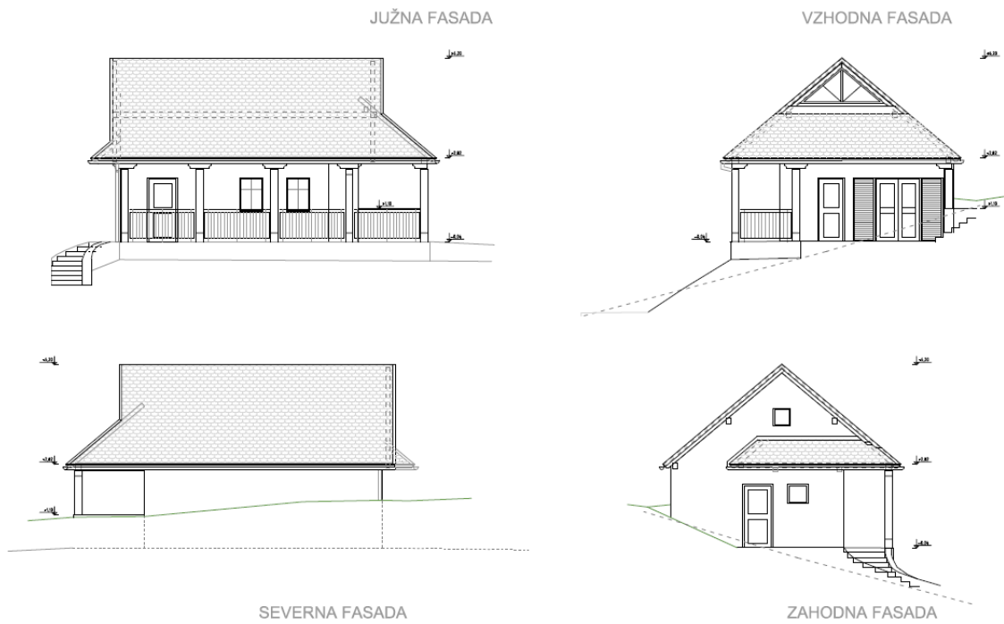
Slika 39: Skica ureditve mrliške vežice Skomarje
