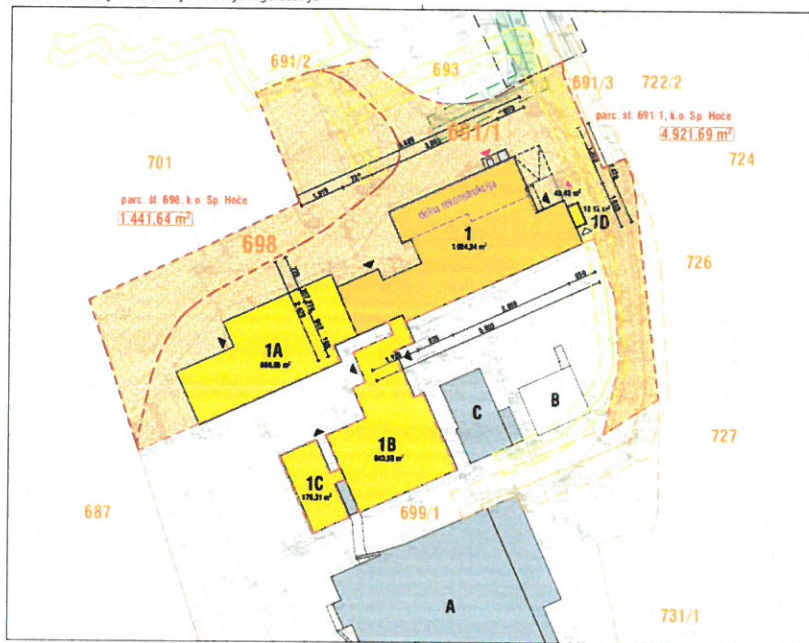
Slika 3-3: Lokacijska situacija obstoječega stanja
