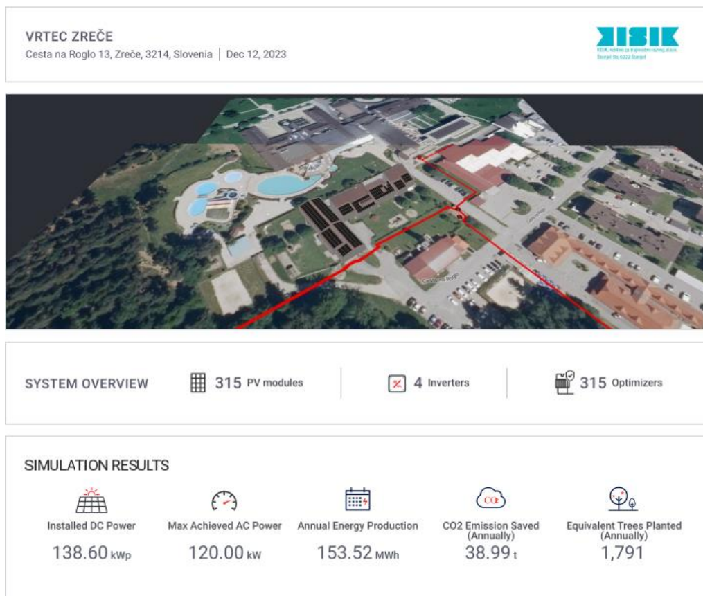
Slika 10: Idejna zasnova sončne elektrarne na stavbi vrca Zreče
