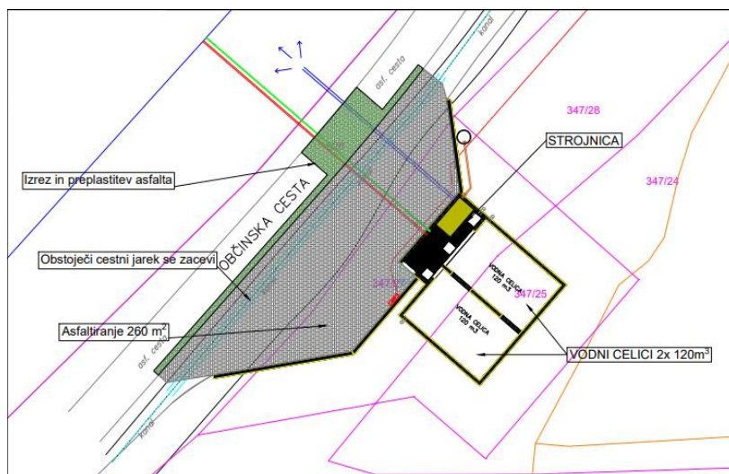
Slika 7: Pregledna situacija vodohrana Križevac
