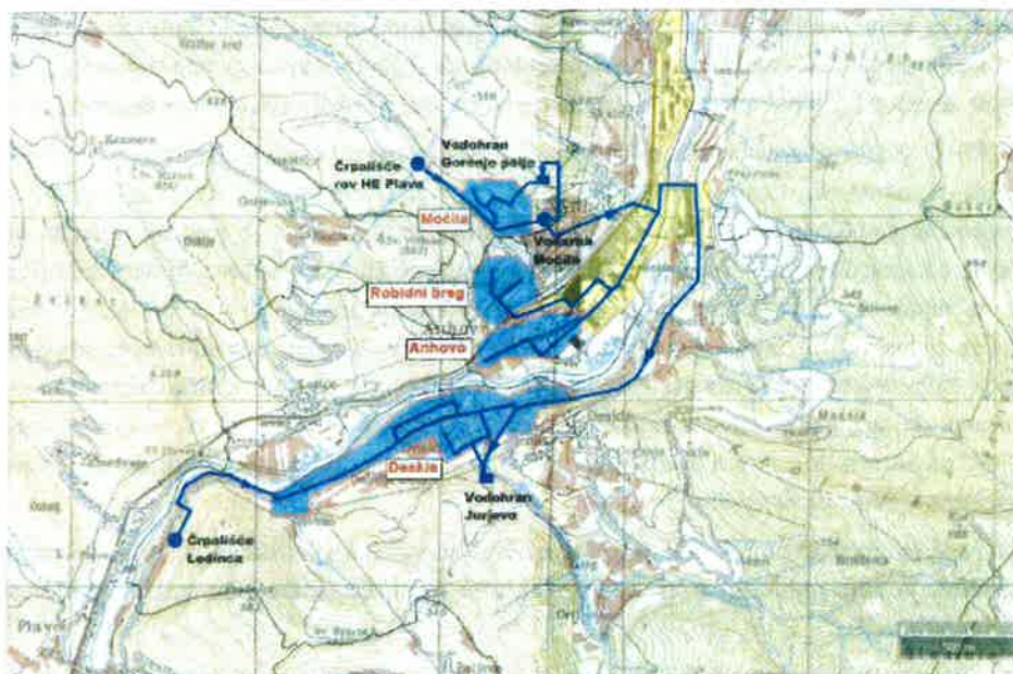
Slika 1 Sistem oskrbe s pitno vodo Deskle–Anhovo
