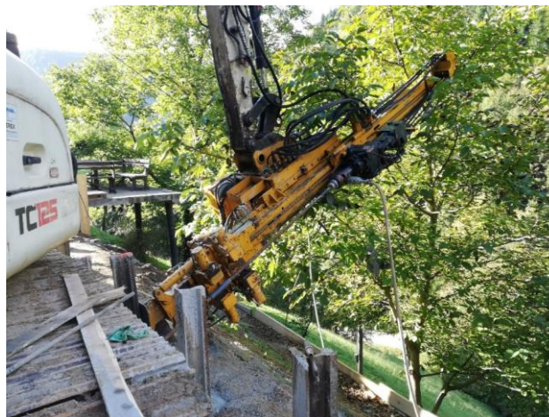
Slika 8: Vrtanje sider
