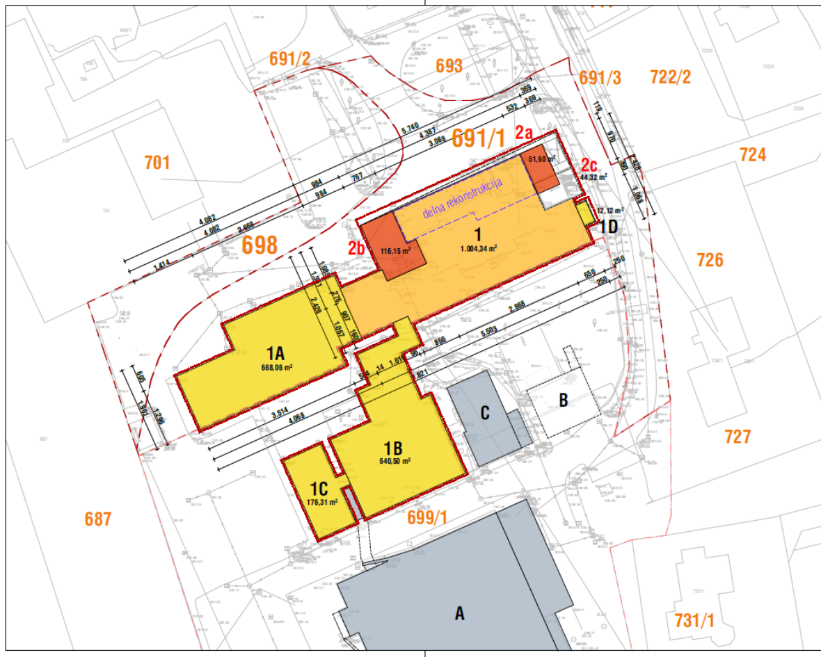
Slika 6-1: Gradbena in ureditvena situacija
