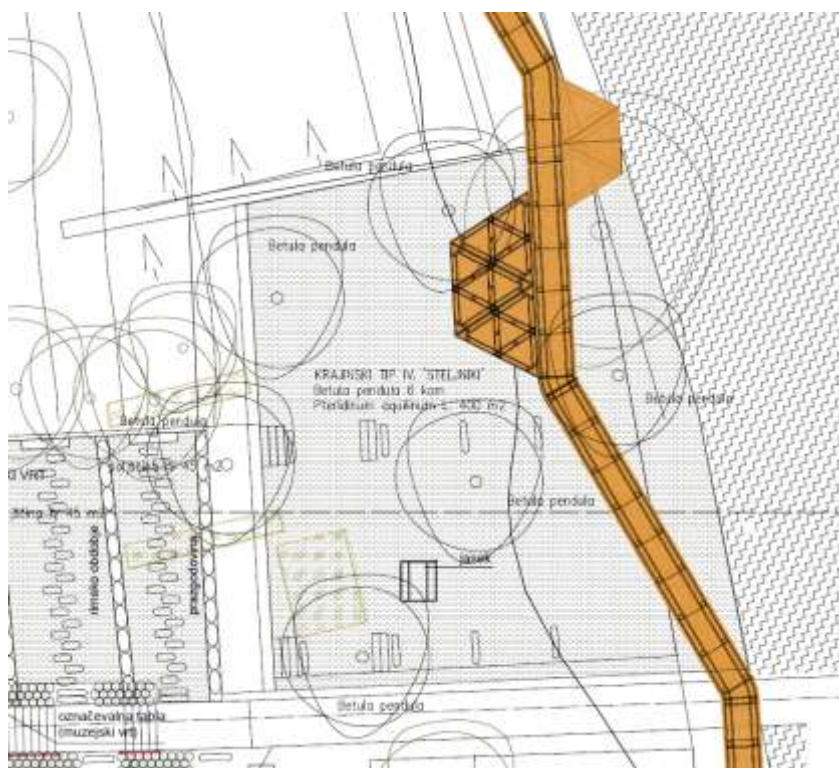
Slika 1: Del ureditve obvodne poti pod Mestno muzejsko zbirko ob mostičku na Majer.
