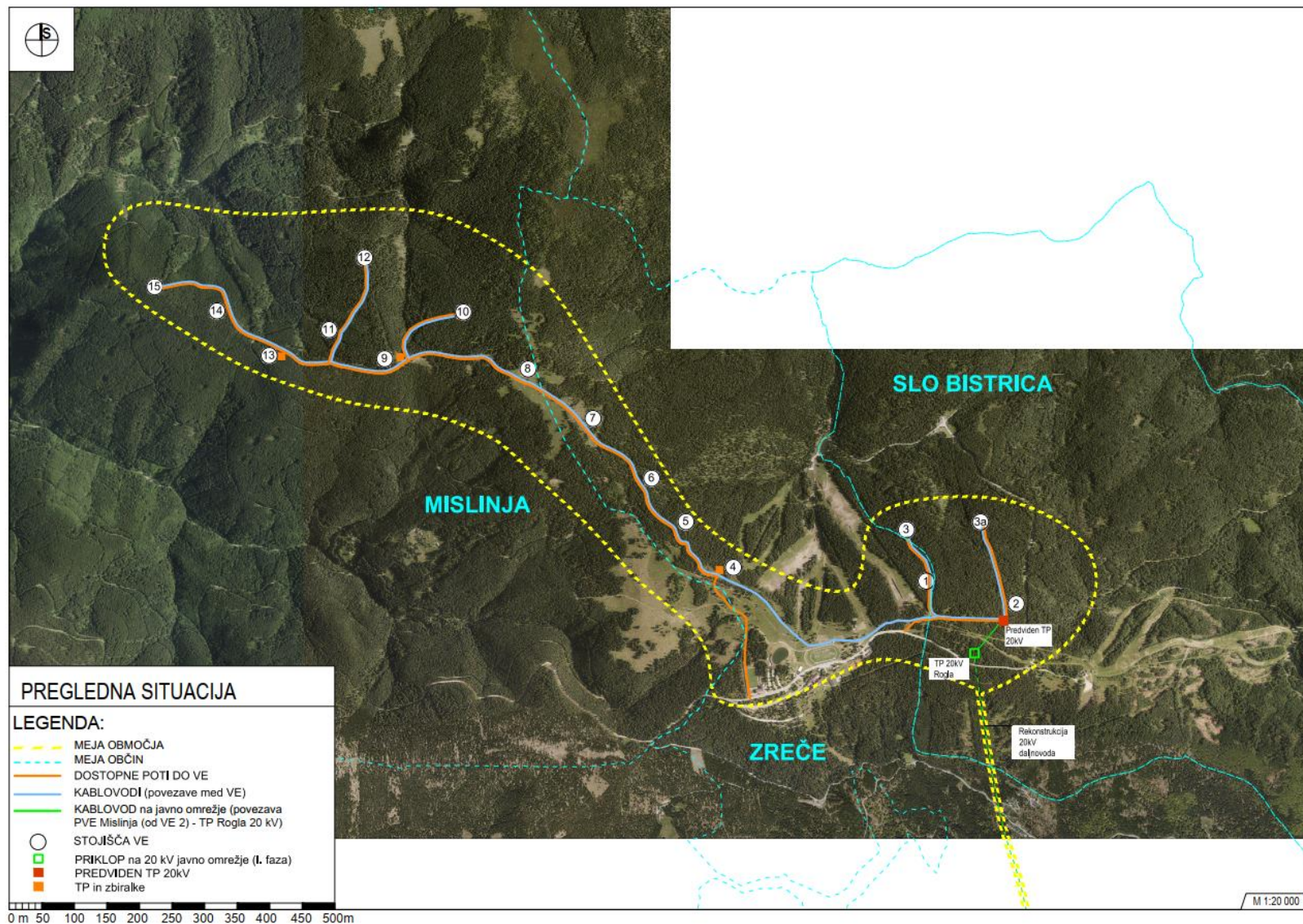
Slika 1: Pregledna situacija postavitve vetrnih elektrarn v Pobudi za DPN vetrne elektrarne Mislinja
