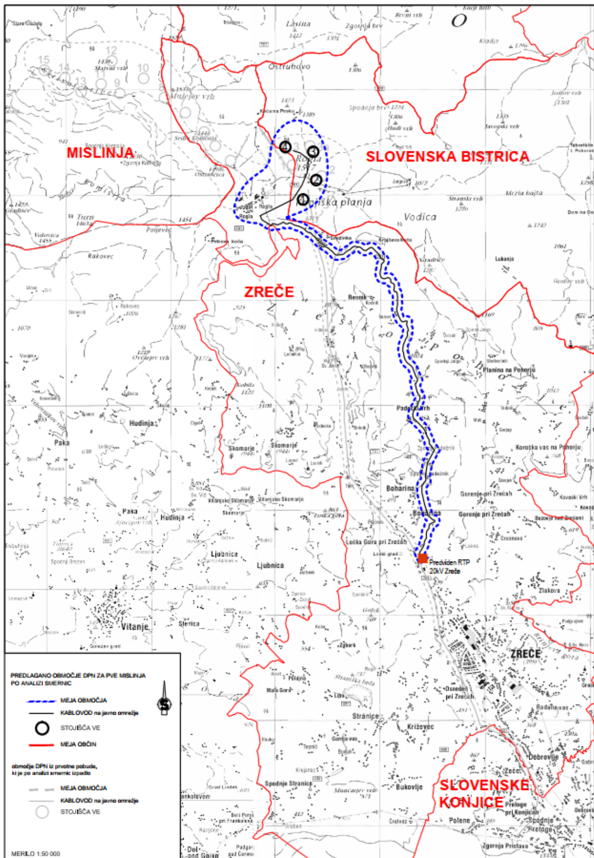
Slika 2: Predlagana stojišča vetrnih elektrarn DPN vetrne elektrarne Mislinja po analizi smernic
