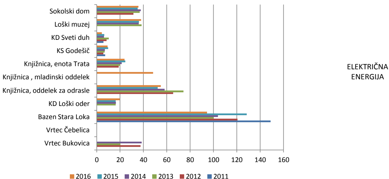
Grafikon 7: Specifična poraba energije(energijsko število) v skupini ostale stavbe v obdobju 2011 – 2016 v kWh/m 2 vir: sistem spremljanja rabe energije (ENEKOM, Inštitut za energetske svetovanj, d.o.o.)
