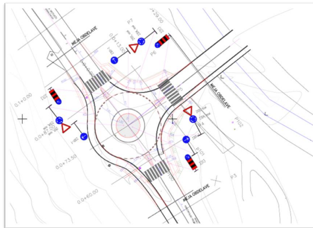
Slika 19: Prometna situacija mini krožišča
