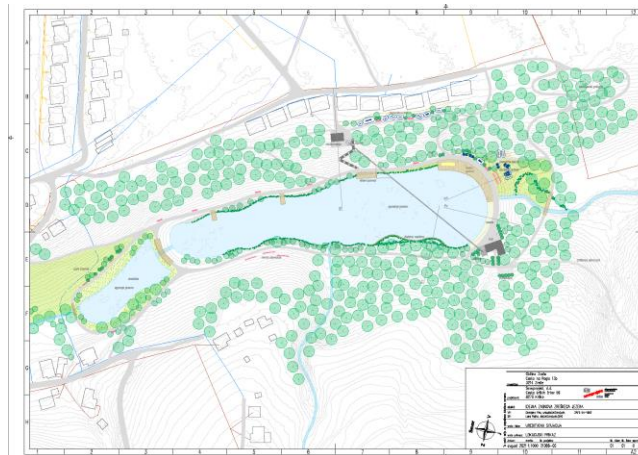
Slika 13: Idejna zasnova ureditve Zreškega jezera
