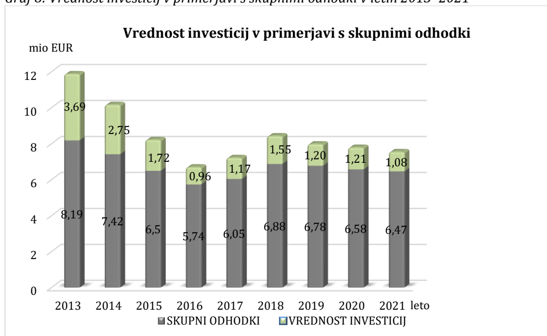
Graf 8: Vrednost investicij v primerjavi s skupnimi odhodki v letih 2013–2021
