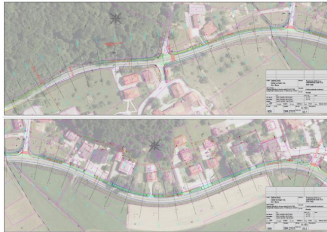
Slika 34: Predvidena rekonstrukcija ceste s pločnikom in kolesarsko stezo Stranice proti Vitanju
