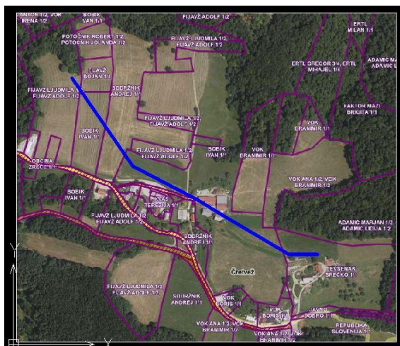
Slika 106: Trasa vodovoda
