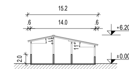
Prezrez A-A
