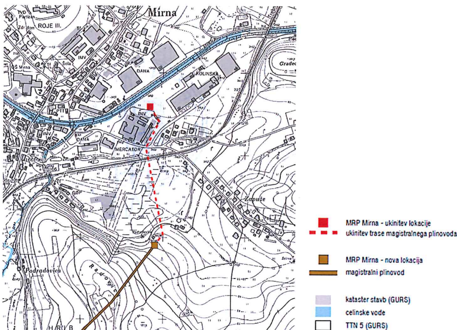
Slika 1: trasa magistralnega plinovoda s prikazano spremembo (vir: GURS).
