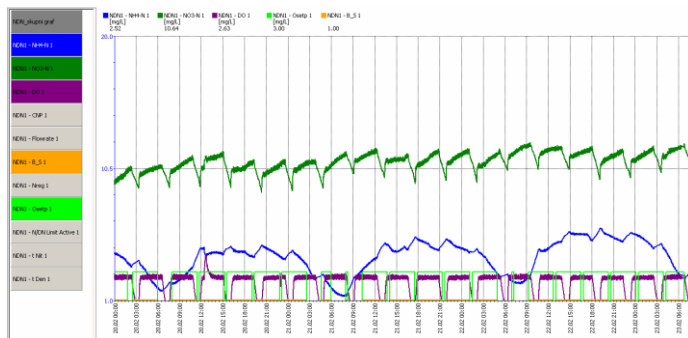
Slika 59: Potek avtomatska nitrifikacija/denitrifikacija
