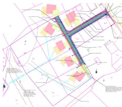
Slika 21: Idejna zasnova projekta
