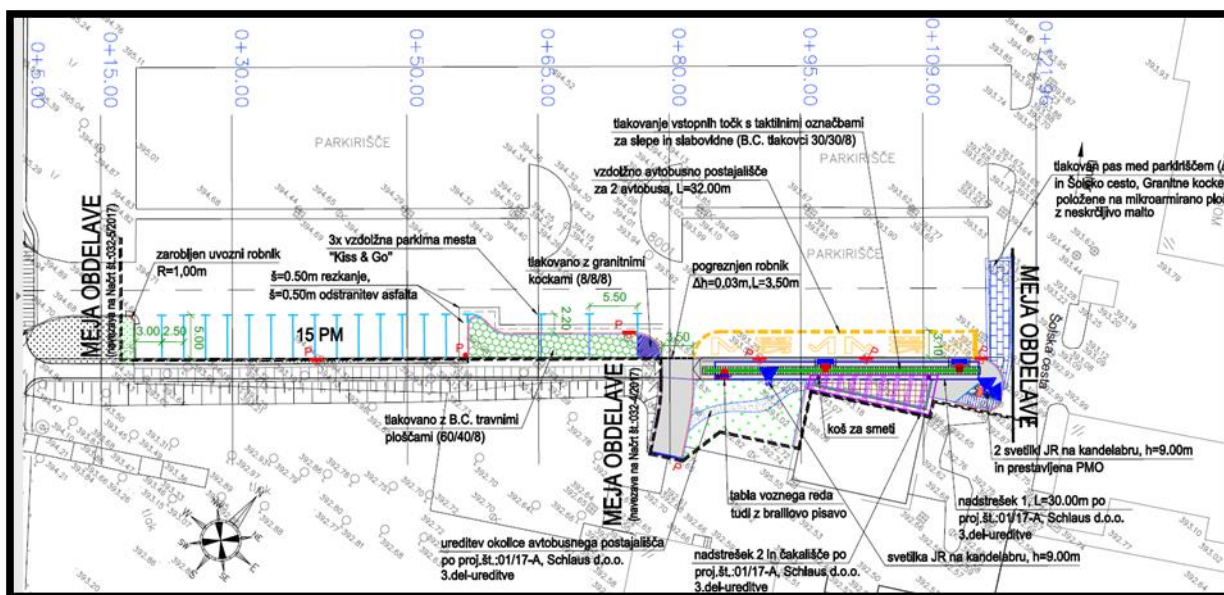
Slika 6: Ureditev avtobusnega postajališča
