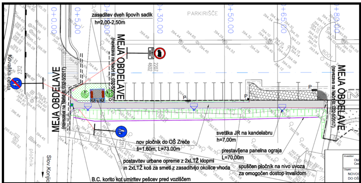
Slika 7: Ureditev pešpoti
