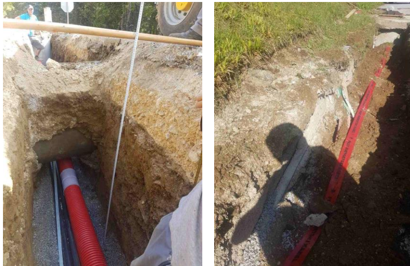
Sliki 24 in 25: Izdelava priključka elektrike
