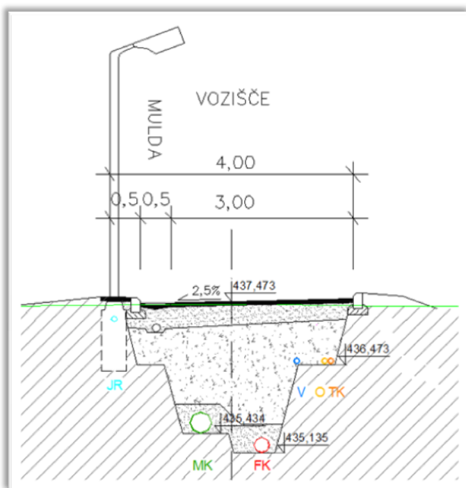
Slika 19: Prečni prerez
