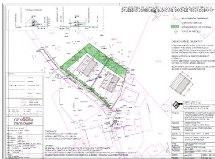
Slika 9: Ureditvena situacija
