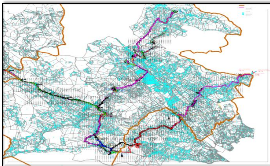
Slika 13: Magistralni vodovod
