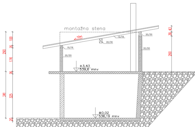
Prečni prerez - novo
