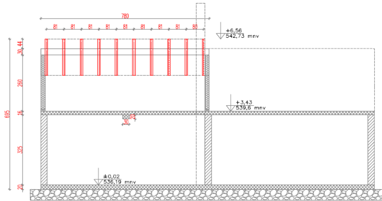
Vzdolžni prerez
