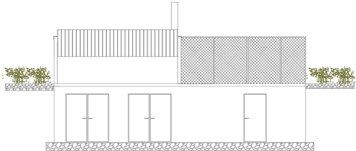
Južna fasada – novo
