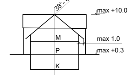
KARAKTERISTIČNI PREREZ OBJEKTA: m 1:500
