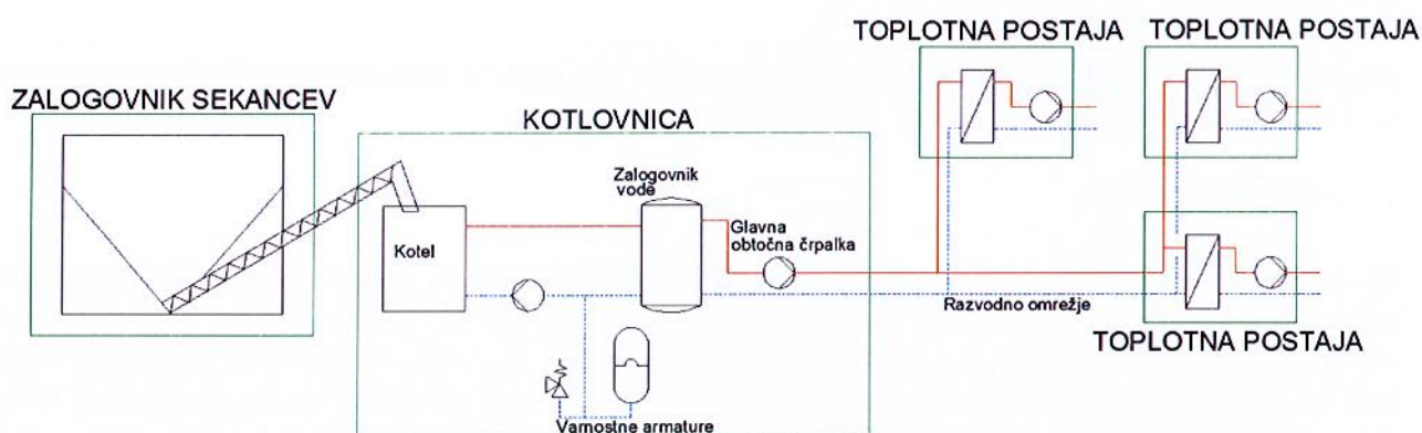
Slika 1: shema DOLB
