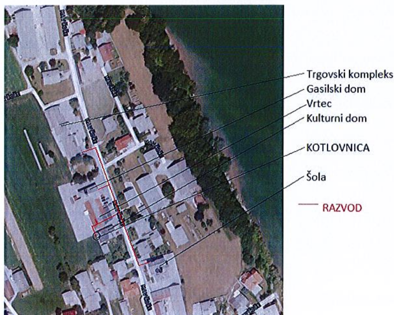
Slika 7: Situacija razvodov
