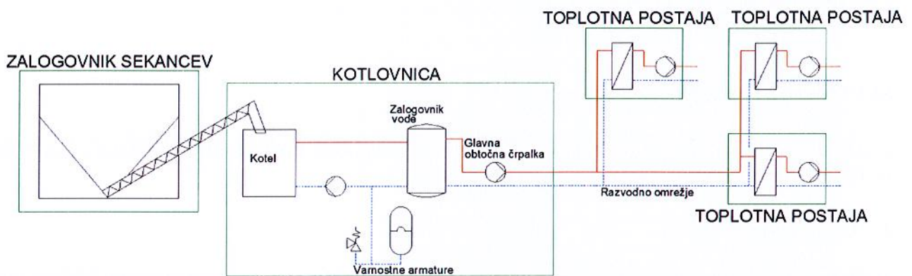
Slika 1: shema DOLB
