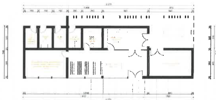
Slika 10: Variantna rešitev tlorisa: 4
