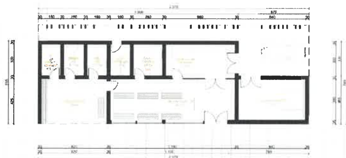
Slika 9: Variantna rešitev tlorisa: 3
