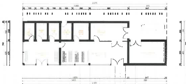
Slika 8: Variantna rešitev tlorisa: 2
