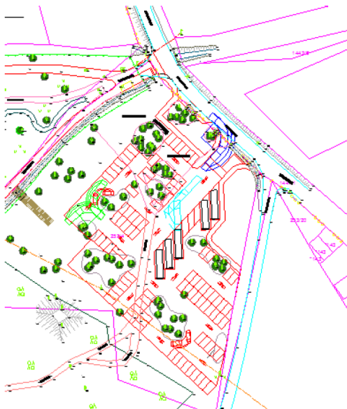
Slika 6: Predlog ureditve parkirišča s prikazom prevoznosti avtobusa ter osebne in dostavne vozila
