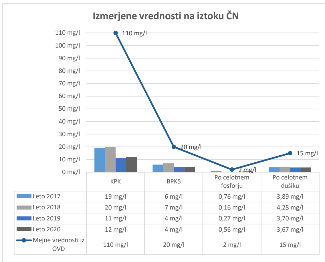
GRAF 2: MEJNE IN IZMERJENE VREDNOSTI NA IZTOKU CENTRALNE ČISTILNE NAPRAVE RAVNE
