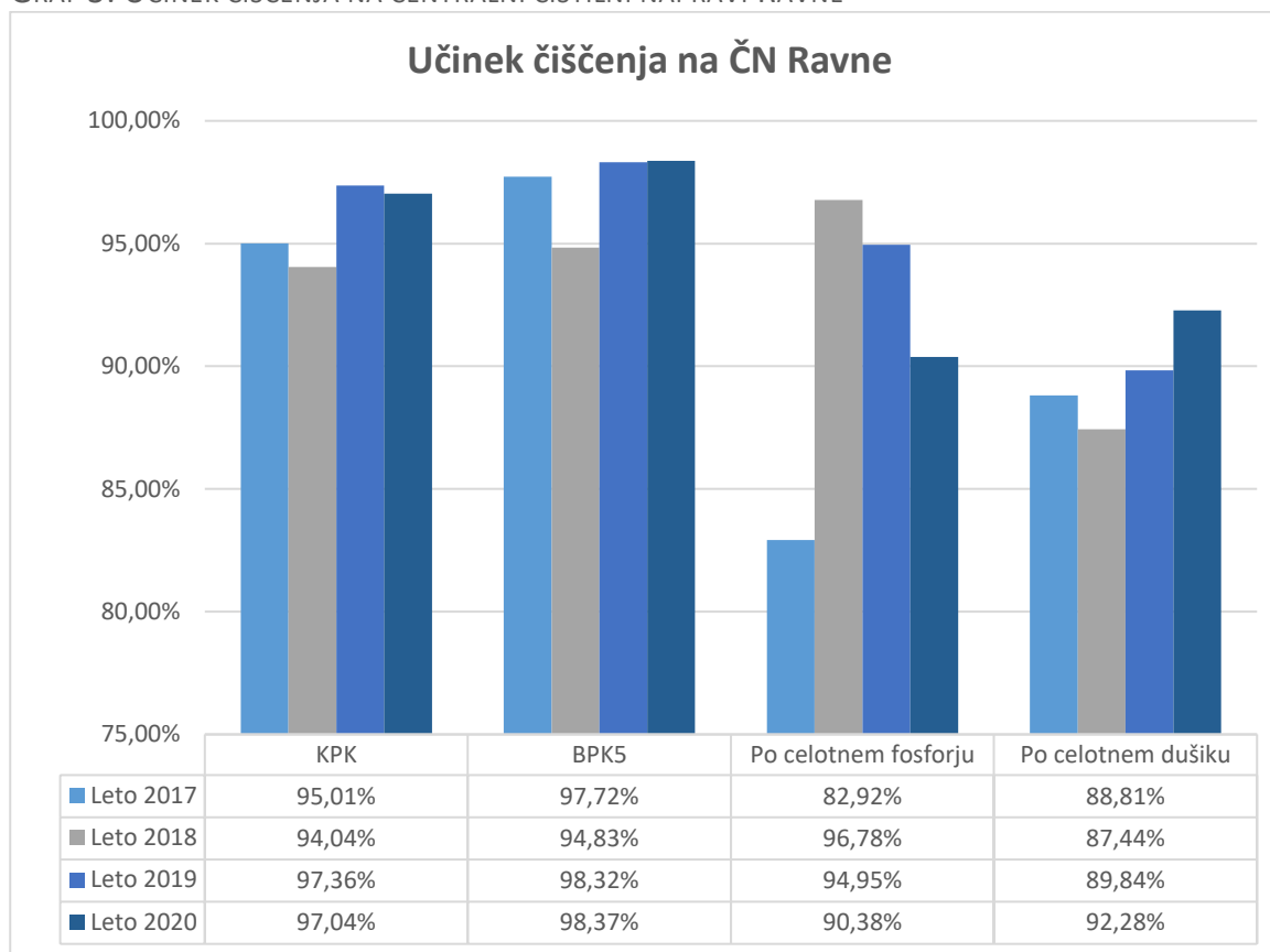
GRAF 3: UČINEK ČIŠČENJA NA CENTRALNI ČISTILNI NAPRAVI RAVNE
