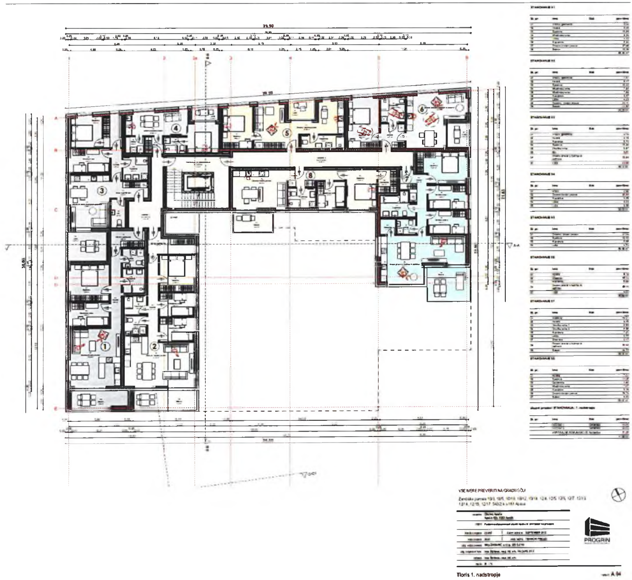
Slika 4: Shema predvidene tlorisne zasnove poslovno-stanovanjskega objekta (zasebni del -I. etaža):
