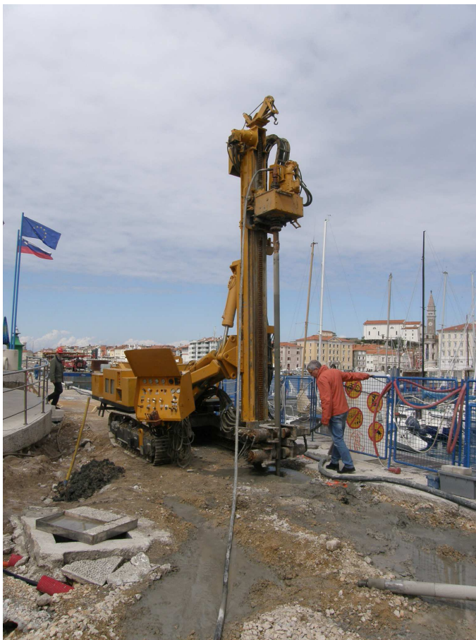
Utrjevanje roba pomola z vbrizgavanje betona.
