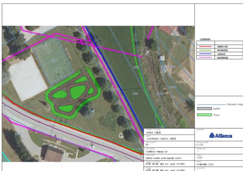
Slika 9: Umestitev poligona v prostor
