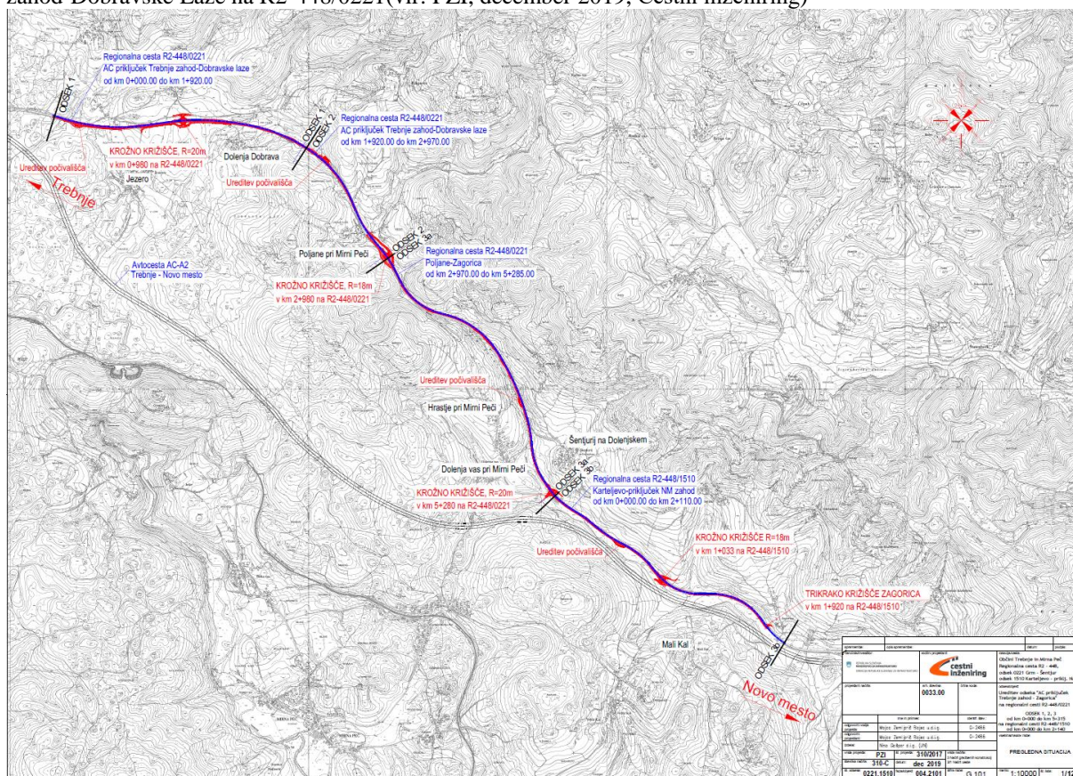
Slika 3: Kolesarske površine, ki jih bo DRSI izvedla v okviru projekta Ureditev odseka AC priključek Trebnje zahod-Dobrovske Laze na R2-448/0221(vir: PZI, december 2019, Cestni inženiring)
